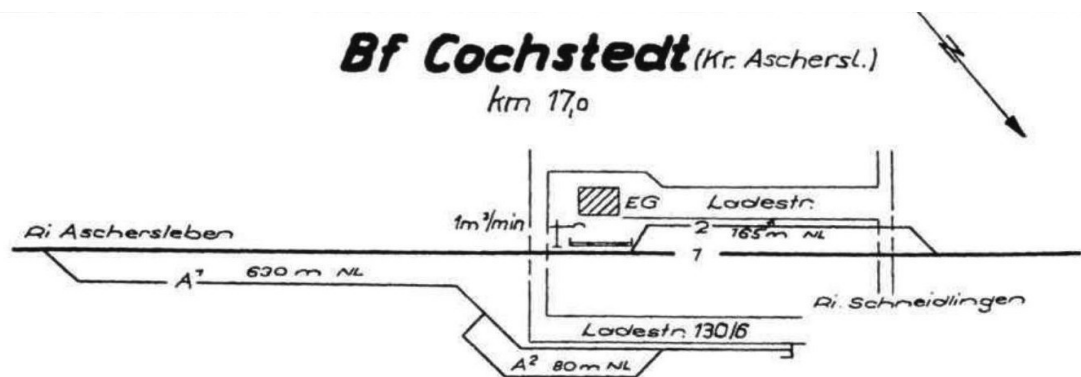
Der Gleisanschluss Cochstedt bei der ASN 1897\ Der Schienenplan des Bhf. Cochstedt\ Ausschnitt H. Bartzack\ public domain\
